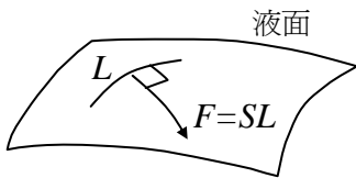
圖 9 與液面平行的張力 F
