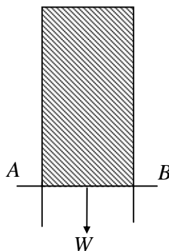
圖 16 液體薄膜與橫桿
