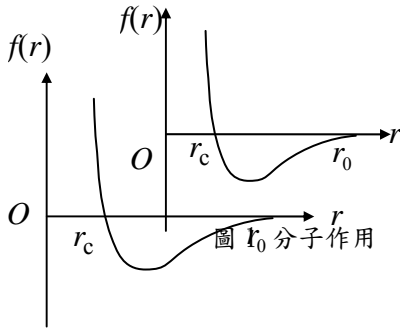
圖 1 分子作用力
