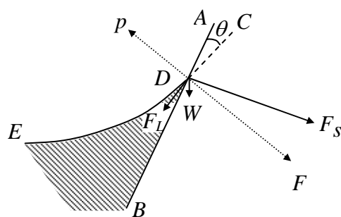
圖 13 液面與管壁接觸處的作用
