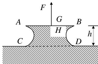
圖 14 上提之長方形平板
