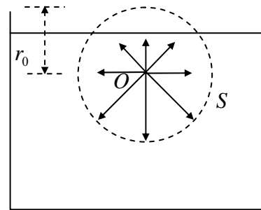
圖 3 液體表面受到的作用力向內
