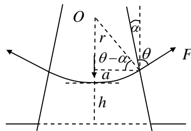
圖 12 錐形液柱的高度
