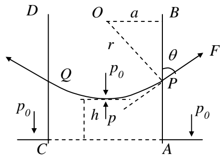
圖 11 毛細管內的液柱高度
