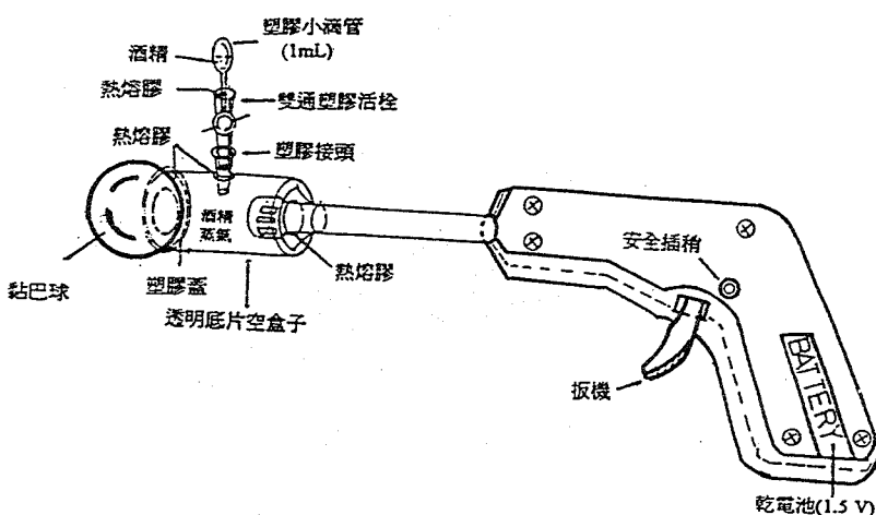
圖 4 新型酒精槍
