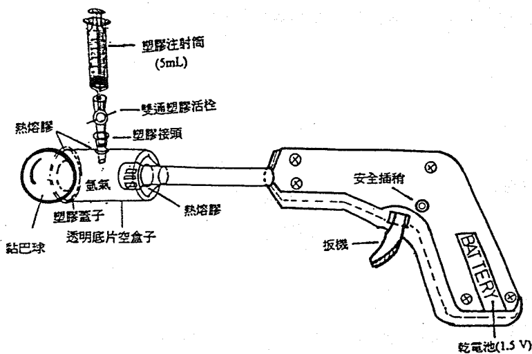
圖 2 新型氫氣槍
