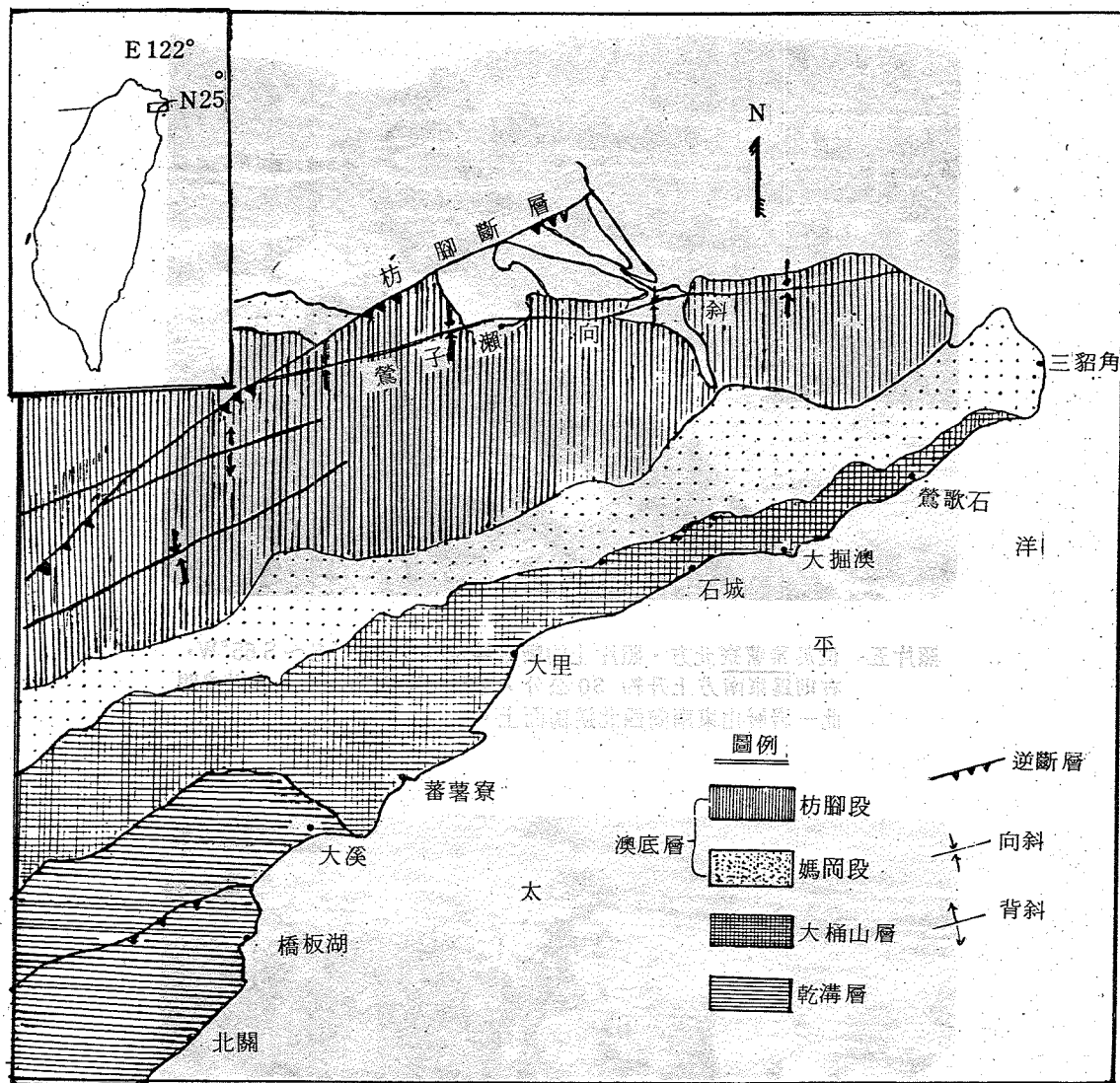
圖一 研究範圍地質圖
