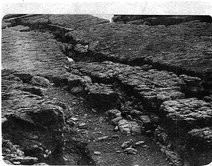
照片二 位於大掘澳附近，在單斜構造的地層斜面上觀察到斷層，屬於平移斷層。
