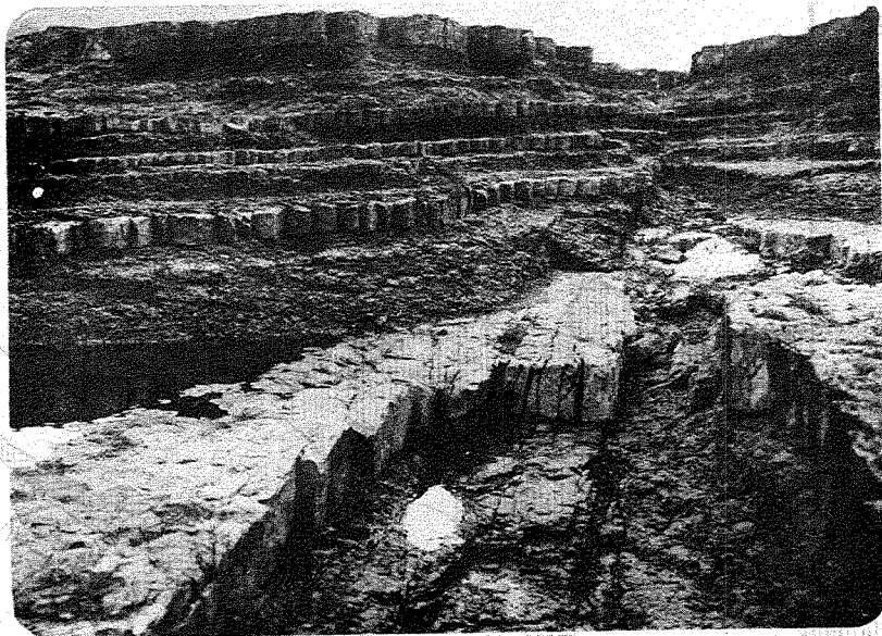
照片五 位於蕃薯寮北方，照片上的斷層線走向為 N65^{\circ}E \sim S65^{\circ}W ，右側為東南方上升約 30 公分，呈現出明顯的對比，可以證明此一岩層由東南向西北逆衝而上。
