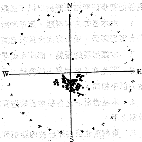
圖三 層態總 Pi 圖
