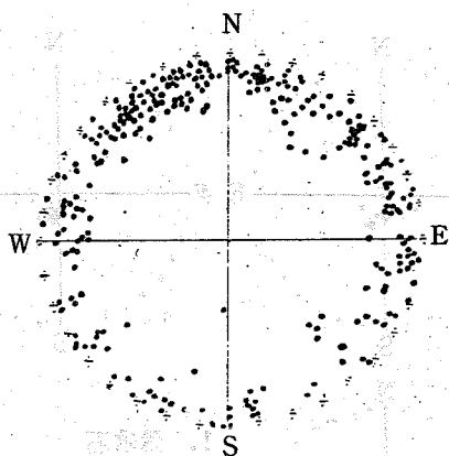
圖四 節理 Pi 圖
