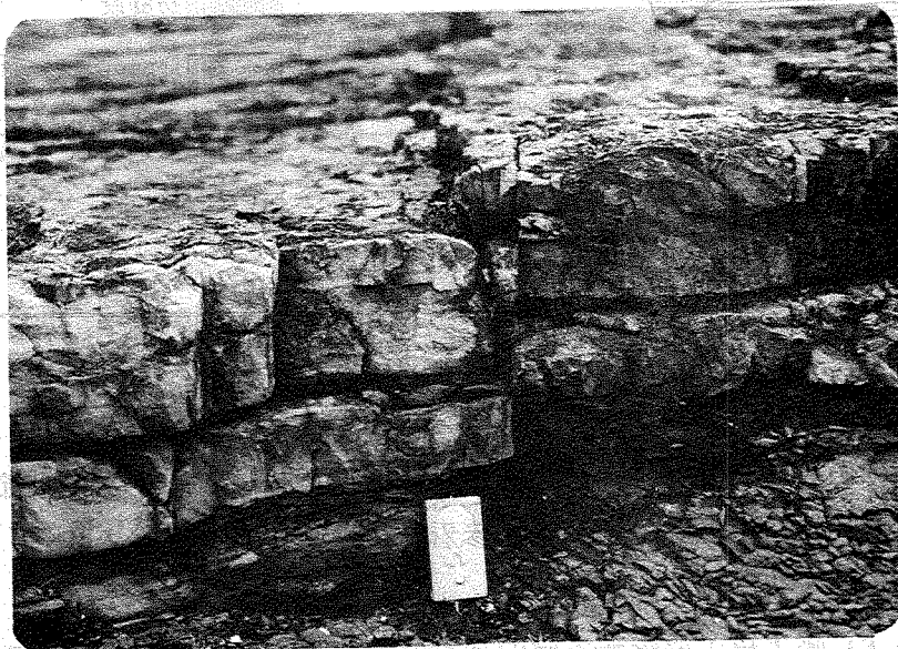
照片六 地點與照片五相同，斷層線走向相同，右側方（東南）明顯上升，上升高度約十多公分。
