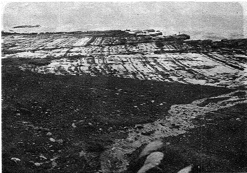
照片一 位於大里陸橋下方波蝕平台上的橫斷層，斷層線與岩層之走向幾乎直角相交。
