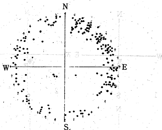
圖五 斷層 Pi 圖
