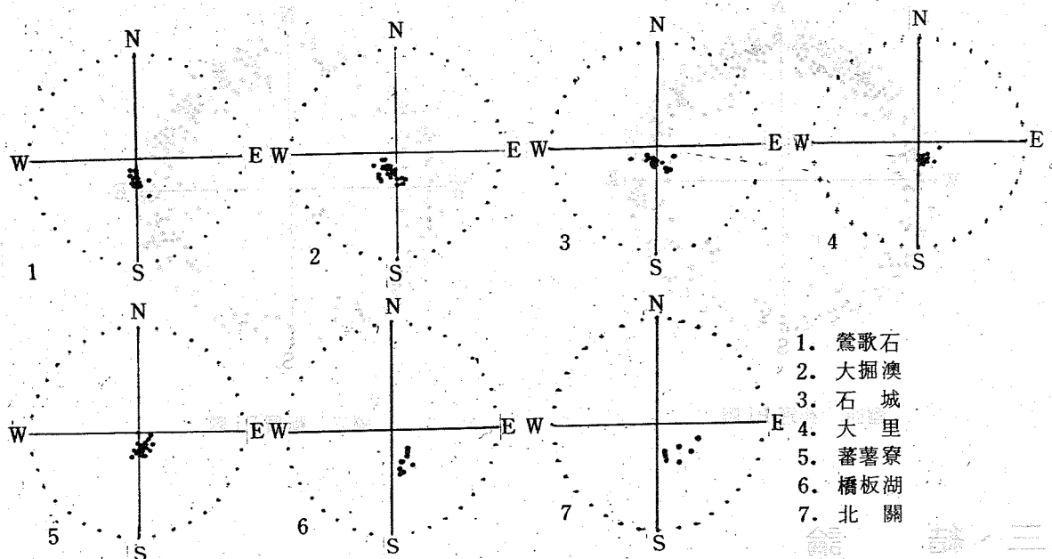
圖二 層態分段 Pi 圖
